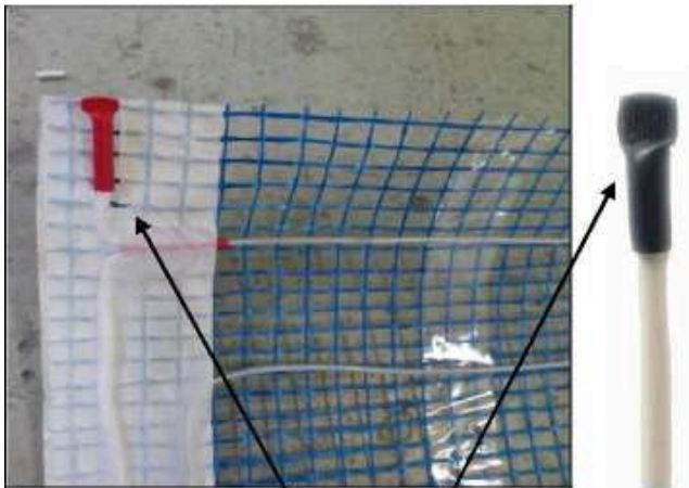
Оконцевание питающего кабеля осуществляется с помощью термоусаживаемой трубки
