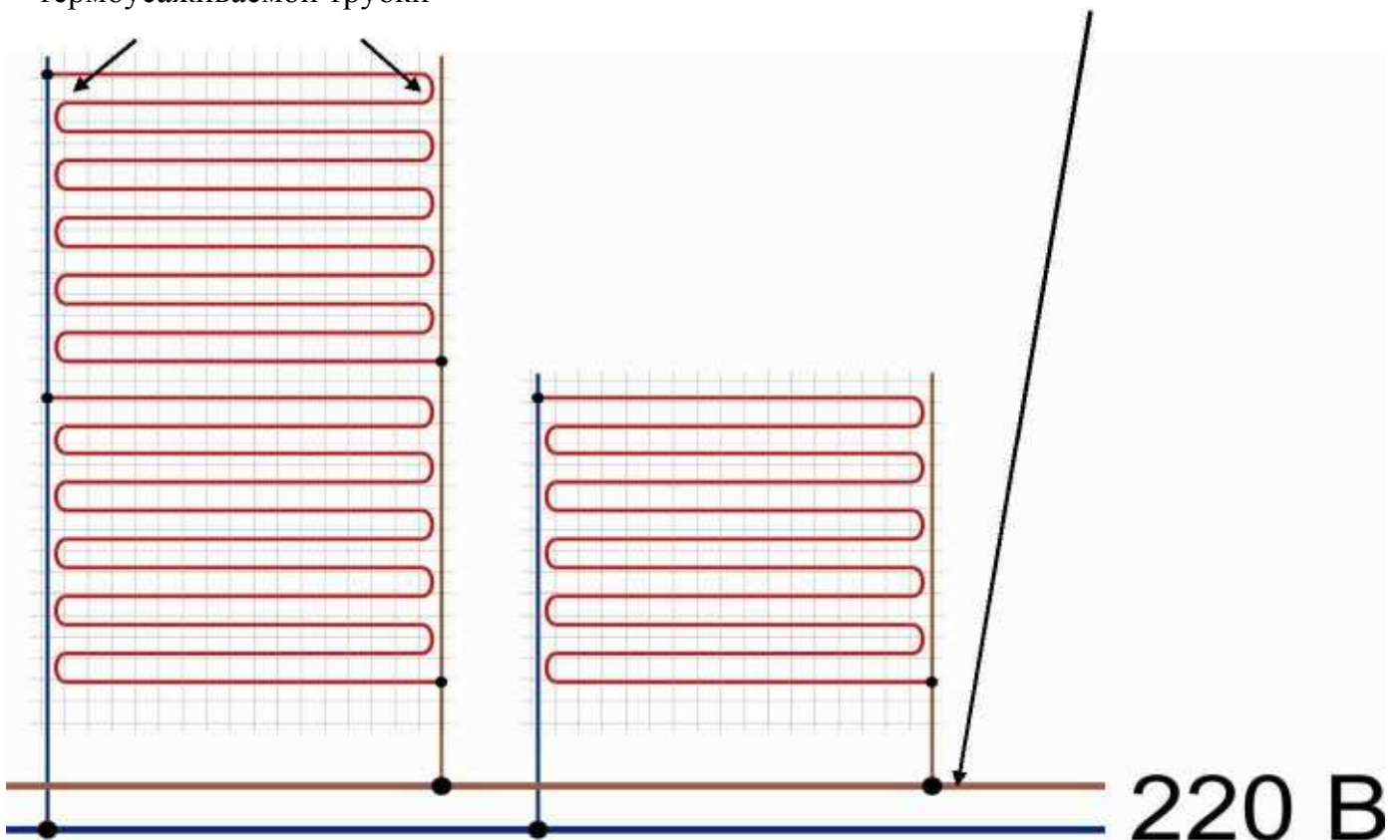
Схема подключения №1
