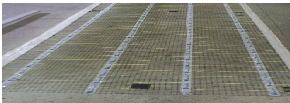
Квадраты битумной ленты
